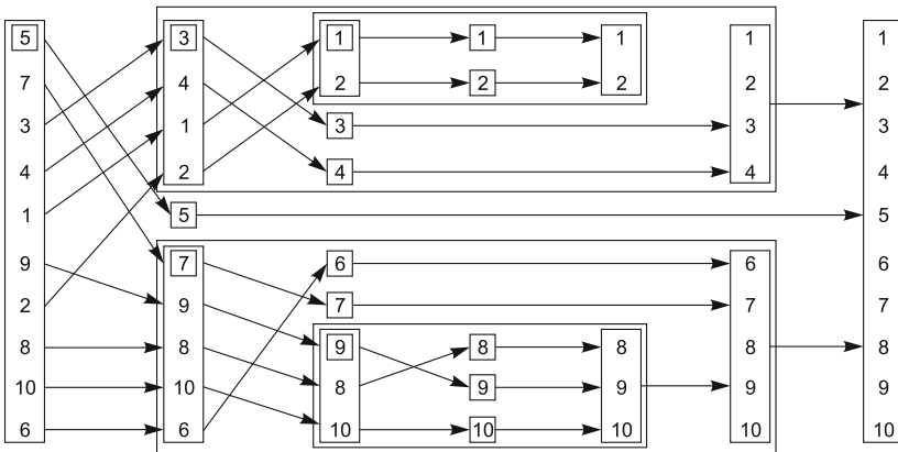
Рис. 4.2. Рекурсивная сортировка в духе ФП
