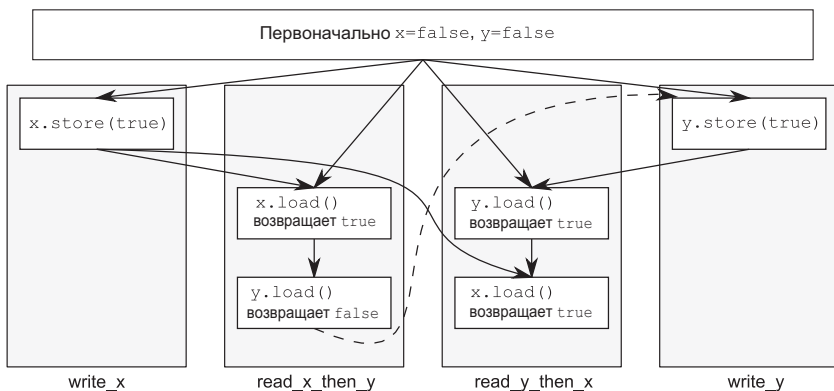
Рис. 5.3. Последовательная согласованность и отношения происходят-раньше
