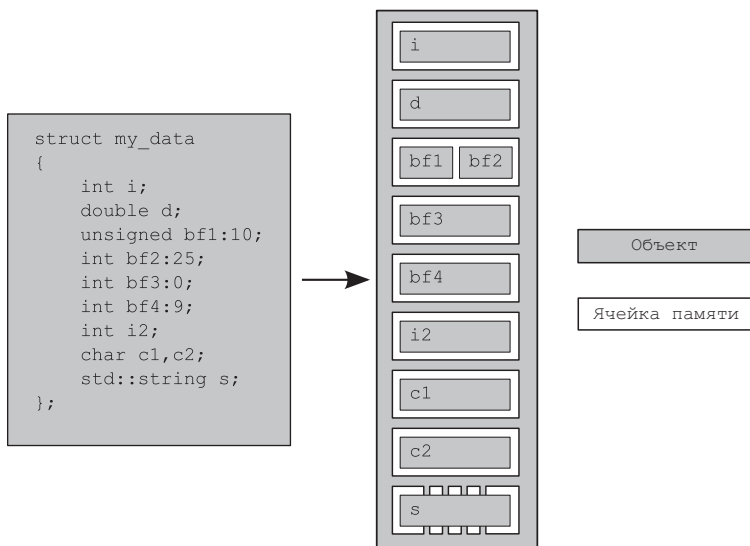
Рис. 5.1. Разбиение struct на объекты и ячейки памяти
