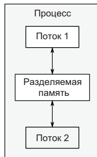
Рис. 1.4. Коммуникация между двумя параллельно исполняемыми потоками в одном процессе
