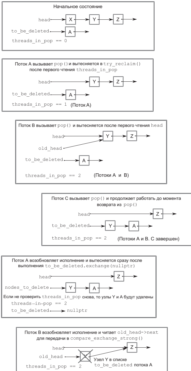
Рис. 7.1. На примере трех потоков, вызывающих pop(), видно, почему необходимо проверять threads_in_pop после заявления прав на список узлов, ожидающих удаления, в try_reclaim()
