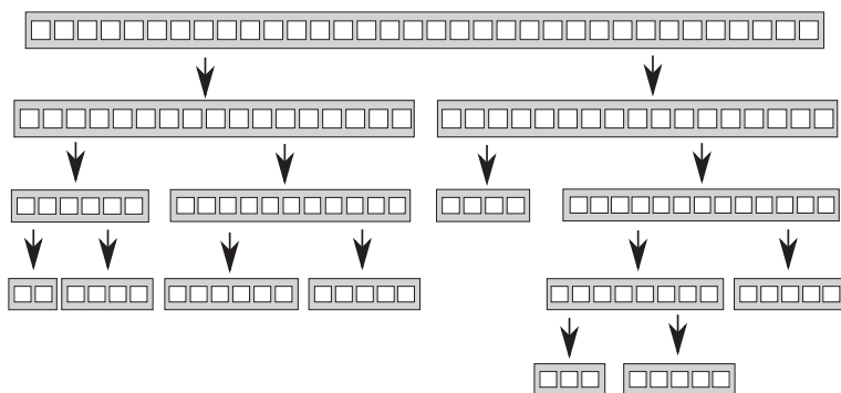
Рис. 8.2. Рекурсивное разбиение данных
