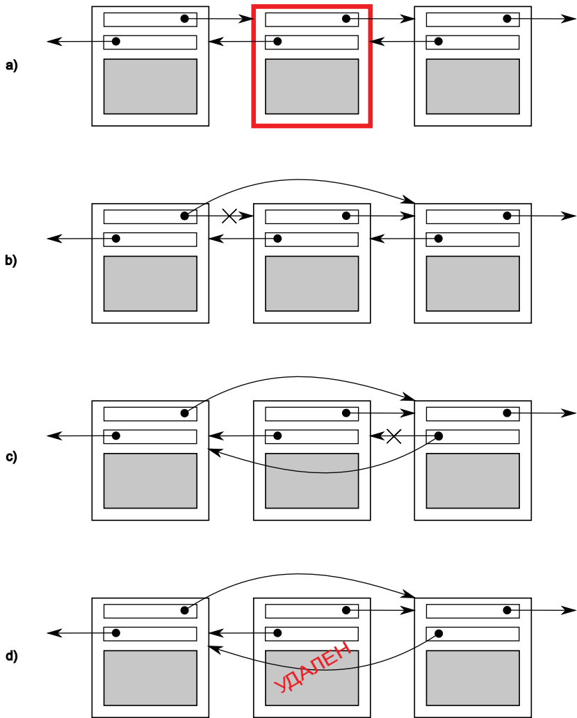
Рис. 3.1. Удаление узла из двусвязного списка
