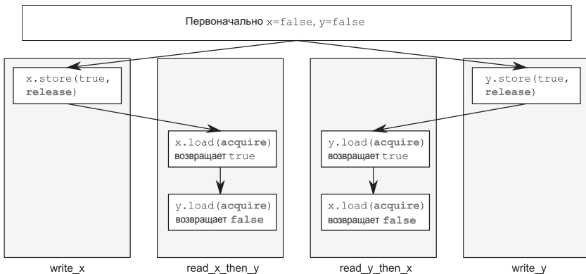
Рис. 5.6. Захват-освобождение и отношения происходит-раньше
