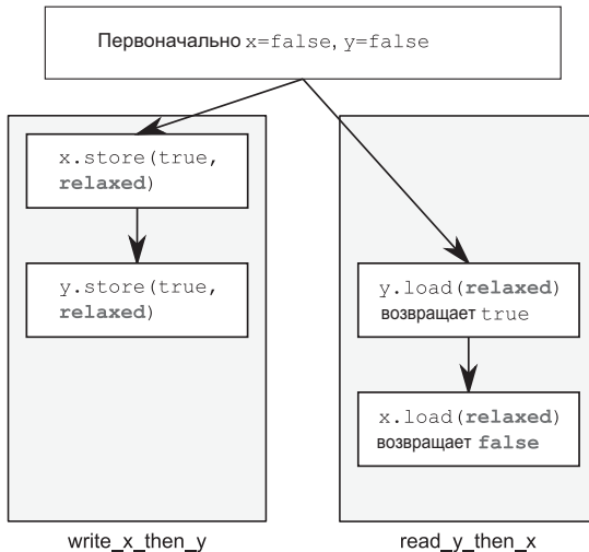
Рис. 5.4. Ослабленные атомарные операции и отношения происходит-раньше
