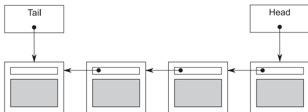
Рис. 6.1. Очередь, представленная в виде односвязного списка
